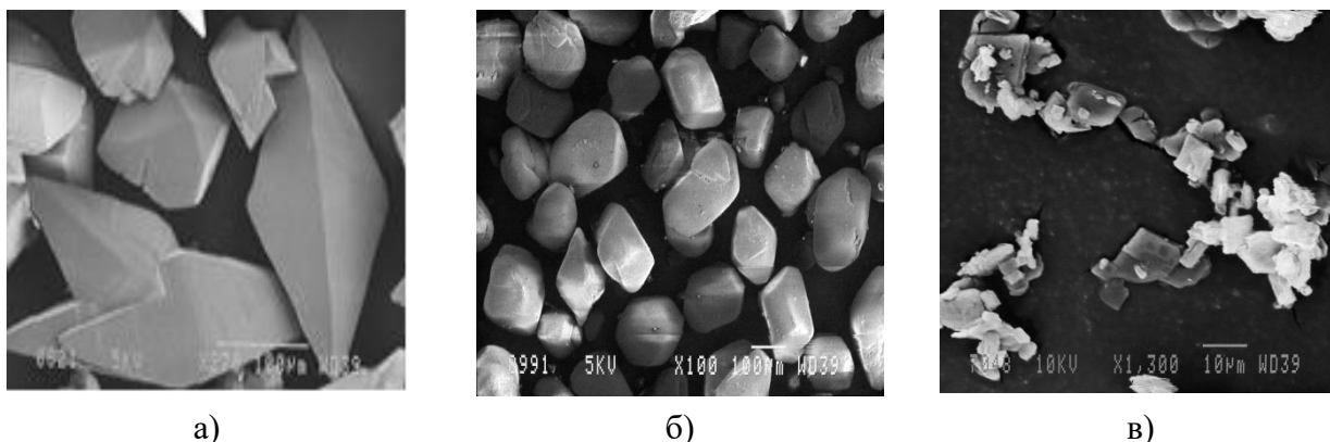
Рисунок 2. Микроструктура типичных образцов а – \epsilon -HNIW, б – \beta -HMX, в – БМК.
