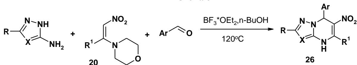
Схема 8
