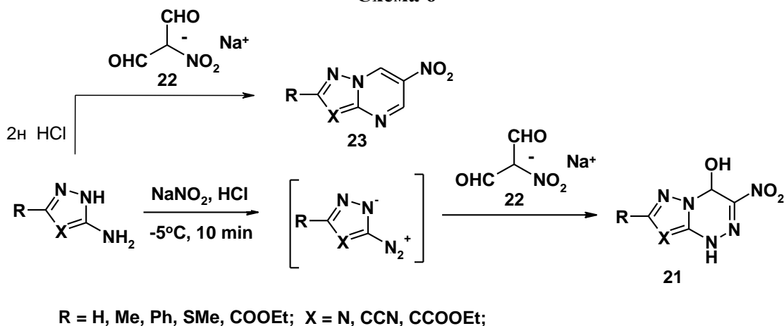
Схема 6
