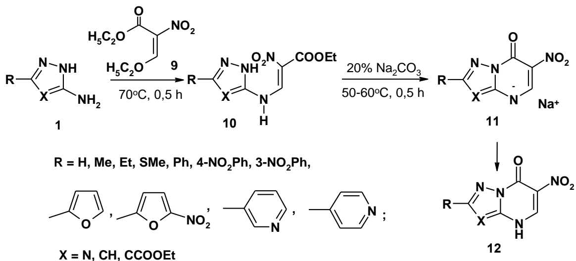
Схема 2
