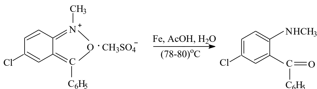
метилсульфат 1-метил-5-хлор-3-фенилантравил
