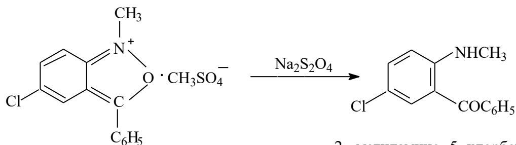
метилсульфат 1- метил-5-хлор-3-фенилантравил
