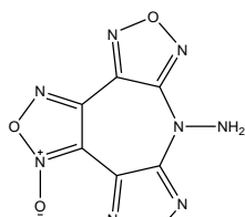
Az(O)NH 2
