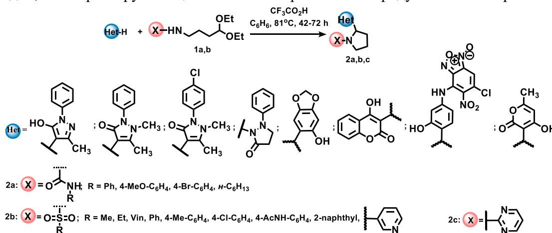
Рисунок 1. Синтез 2-(гетеро)арилпирролидинов
