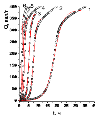
Рисунок 2. Зависимости тепла Q_t , выделившегося при разложении топлива, от времени t при различных температурах: 1 – 161,6; 2 – 171,2; 3 - 175,0; 4 - 180,3; 5 - 184,2; 6 - 188,4; 7 – 198,8°C; точки - эксперимент, сплошные кривые - расчет по уравнению (1).
