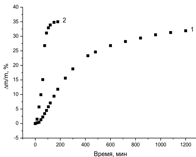
Рисунок 4. Кинетика потери массы при термическом разложении I в 5%-ном растворе динонилфталата (1) и в расплаве (2) при 120°C.
