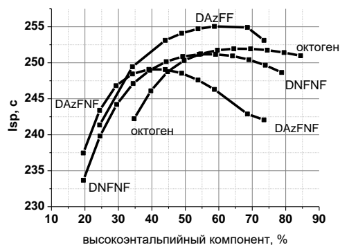
Рисунок 2. Величины I_{sp} композиций 19 об.% АС + высокоэнтальпийный наполнитель + ПХА до 100%.
