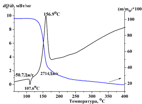
Рисунок 3. Кривые ДСК и ТГ для II при скорости нагрева 5 °C/мин.
