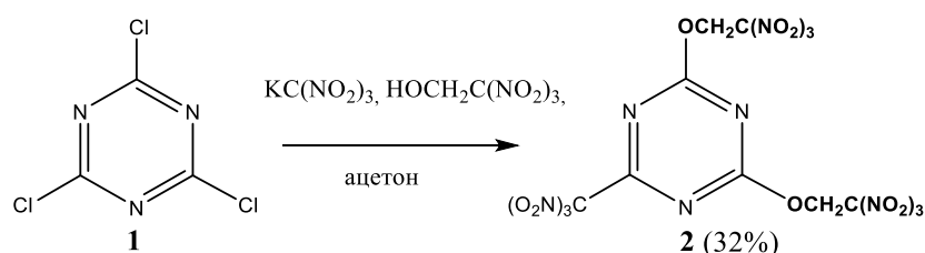
Схема 1
