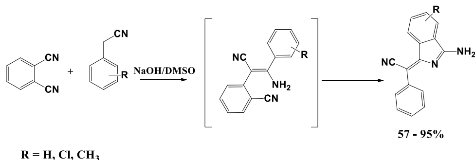
Схема 4. Взаимодействие фталонитрила с арилацетонитрилами
