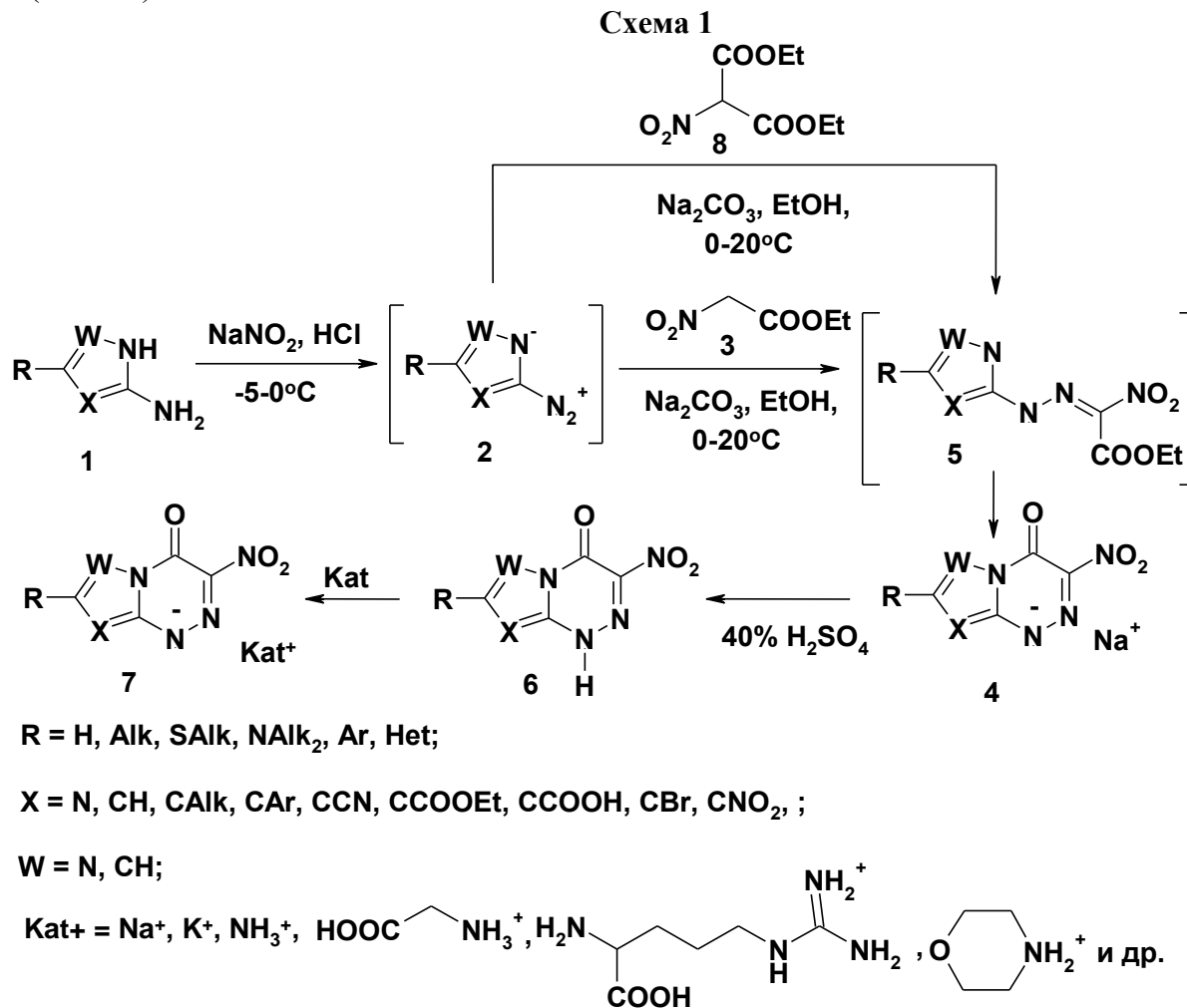
Схема 2
