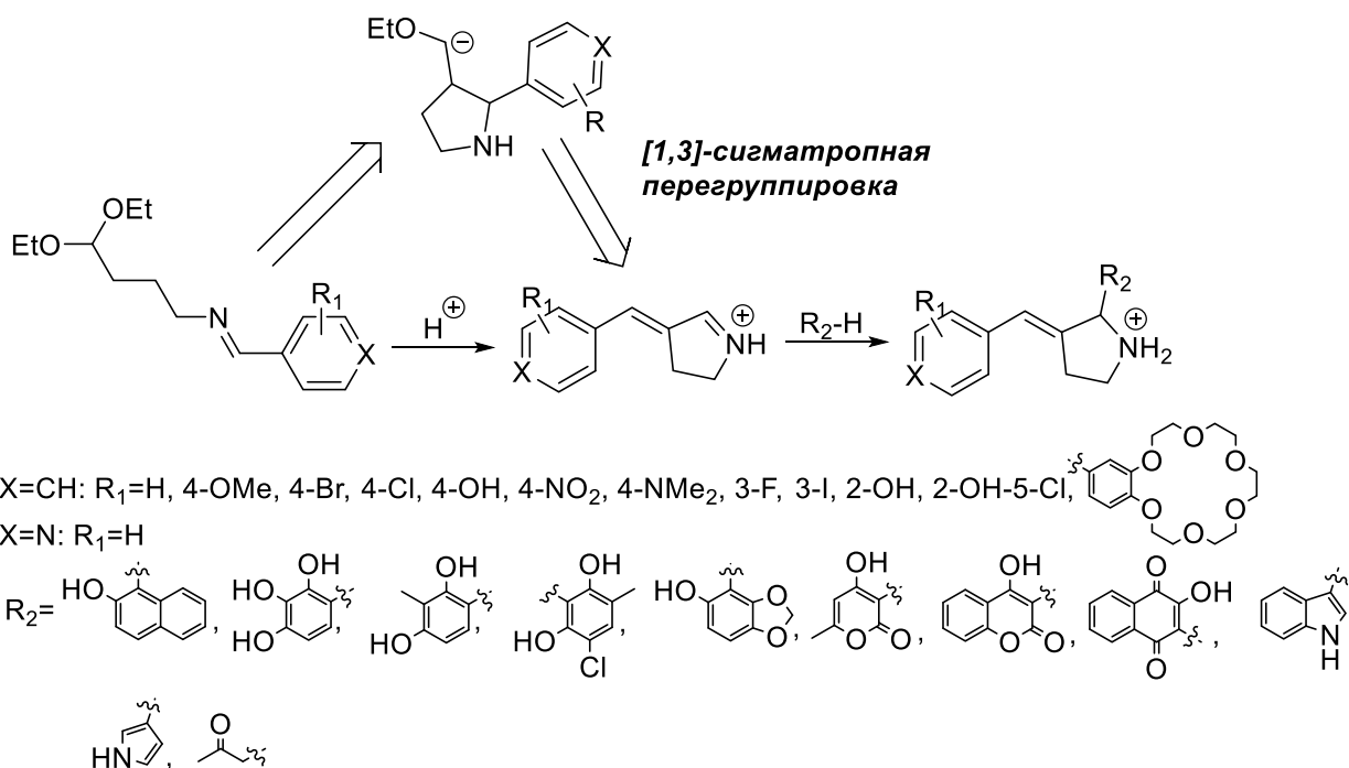
Рисунок 1. Синтез 3-арилиден-1-пирролинов и их взаимодействие с C-нуклеофилами
