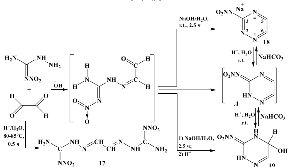
Схема 5
