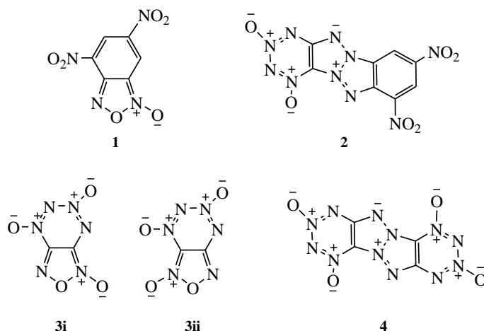
Рисунок 1. Исследуемые соединения 1 - 4.
