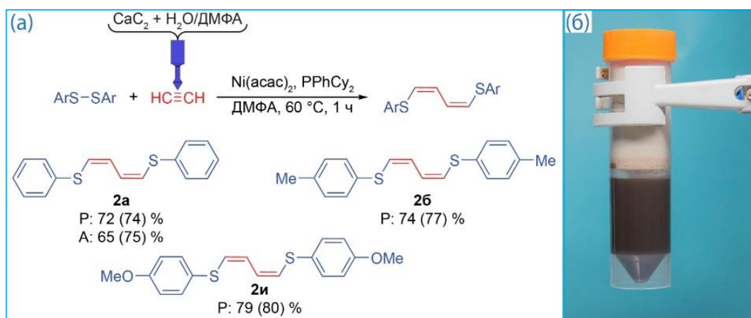
Схема 9. Синтез 1,4-бис(арилтио)бутадиенов-1,3 с использованием ПП реактора: а) продукты реакции (Р – реактор, А – ацетилен из баллона); б) схема реакционной установки.
