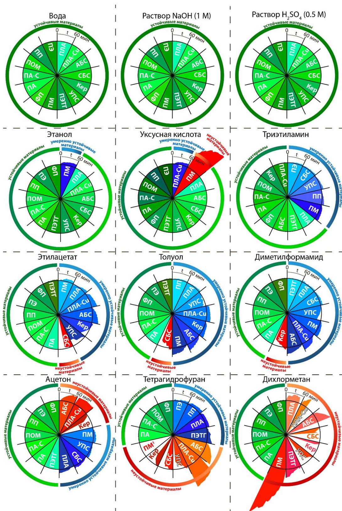
Рисунок 5. Круговые диаграммы изменения площади FFF-изделия под воздействием растворителей в течение 1 ч: (● – красный цвет ) материал разрушается в ходе эксперимента ( \Delta S > 20 \% ); (● – синий цвет ) материал проявляет умеренную устойчивость в ходе эксперимента ( \Delta S = 2 - 20 \% ); (● – зеленый цвет ) материал устойчив в ходе эксперимента ( \Delta S < 2 \% ).
