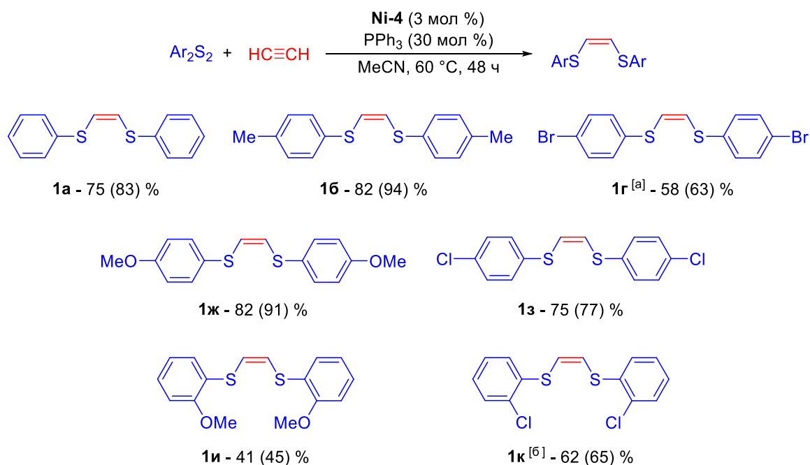
Схема 6. Синтез 1,2-бис(арилтио)этинов с использованием МОК Ni-4 .
