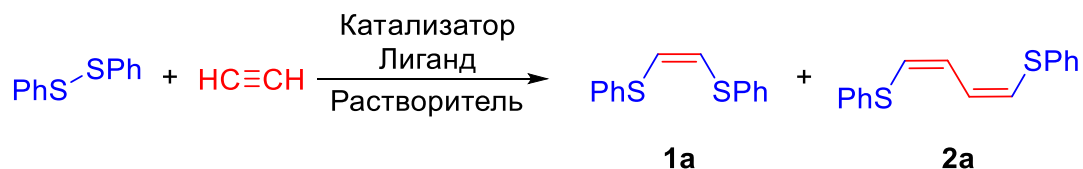
Схема 2. Модельная реакция присоединения дифенилдисульфида к ацетилену.
