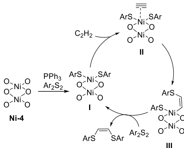
Схема 7. Предполагаемый механизм реакции присоединения диарилдисульфидов к ацетилену, катализируемой МОК Ni-4 .
