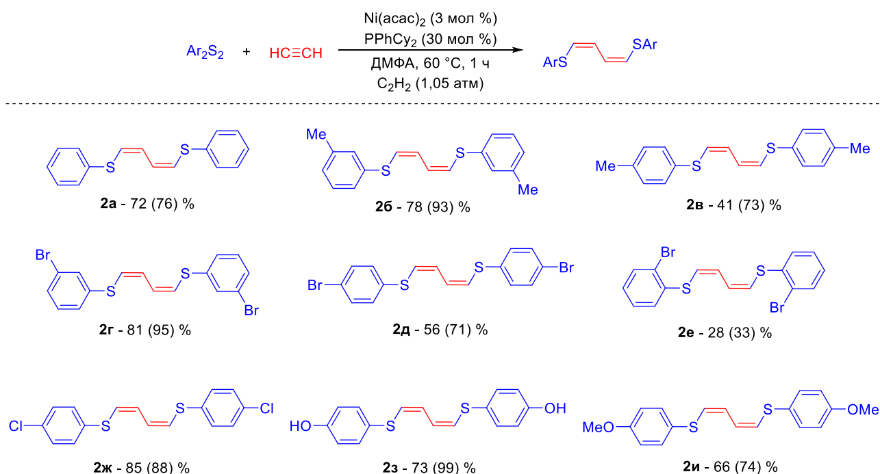
Схема 4. Синтез 1,4-бис(арилтио)бутадиенов-1,3.
