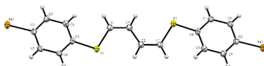
Рисунок 2. Структура соединения 2д , подтвержденная методом РСА.
