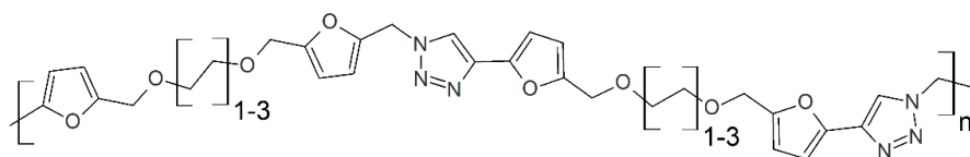
Рис. 1. Получаемый полимер из новых фурановых мономеров, содержащих подвижные этиленовый, бутиленовый и гексиленовый сегменты.
