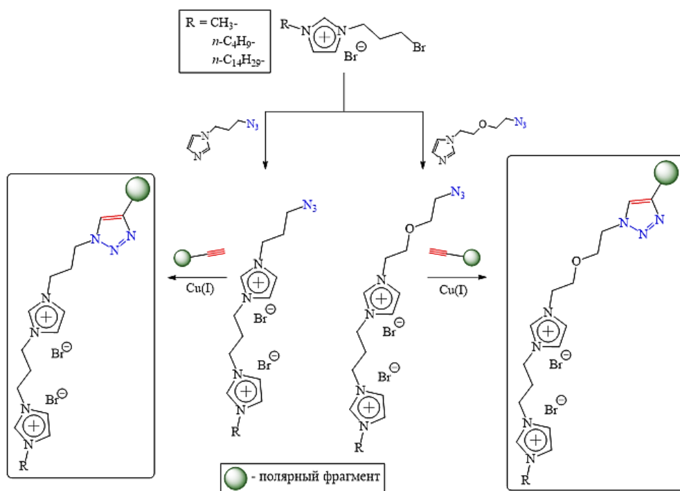
Рис. 1. Получение триазол-содержащих солей бис-имидазолия.
