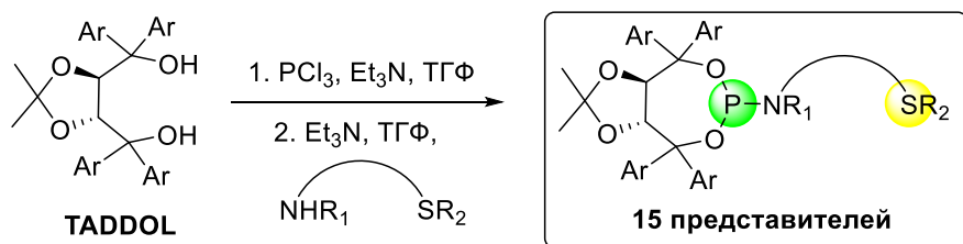
Рис. 1. Синтез лигандов.
