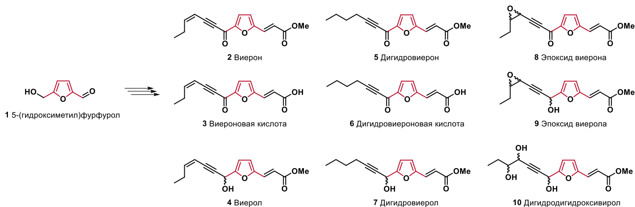
Рис. 1. Соединения виеронового ряда.
