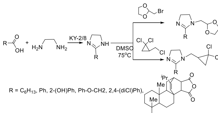
Рис. 1. Схема синтеза 2-замещенных 4,5-дигидро-1Н-имидазолов.
