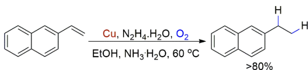
Рис. 1. Реакция восстановления олефинов гидразингидратом.
