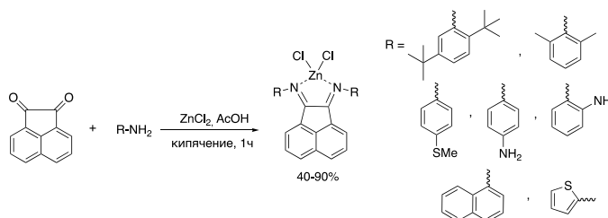
Рис. 3. Синтез Zn-BIAN комплексов.
