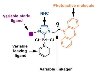
Рис. 1. Общая схема полученных фотоактивных комплексов M/NHC.
