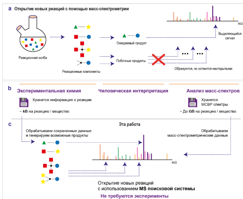
Рис. 1. Открытие новых превращений с помощью автоматического скрининга существующей масс-спектрометрической базы масс-спектров.
