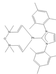
Рис. 2. Структура комплекса 2.
