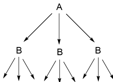
Схема 1. Каталитическая система, не описываемая в терминах TON и TOF.
