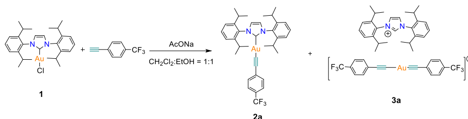
Рис. 2. Изучение реакции получения комплексов NHC/Au (I).
