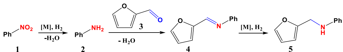
Рис. 1. Восстановительное аминирование фурфурола нитробензолом
