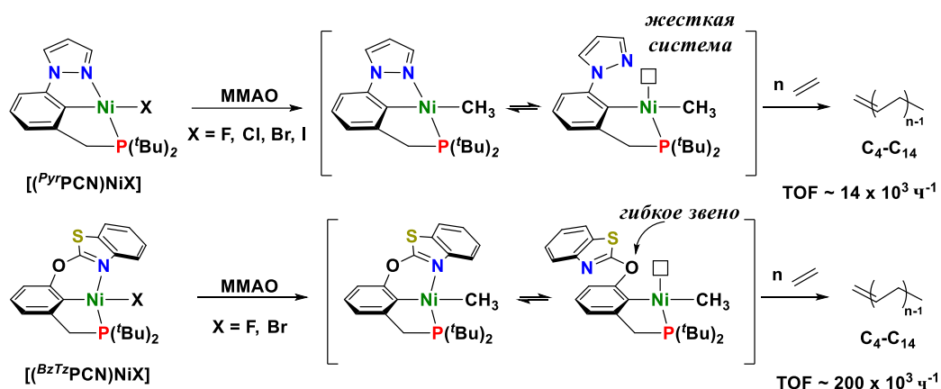
Рис. 1. Несимметричные PCN пинцерные комплексы никеля(II) в процессе олигомеризации этилена.
