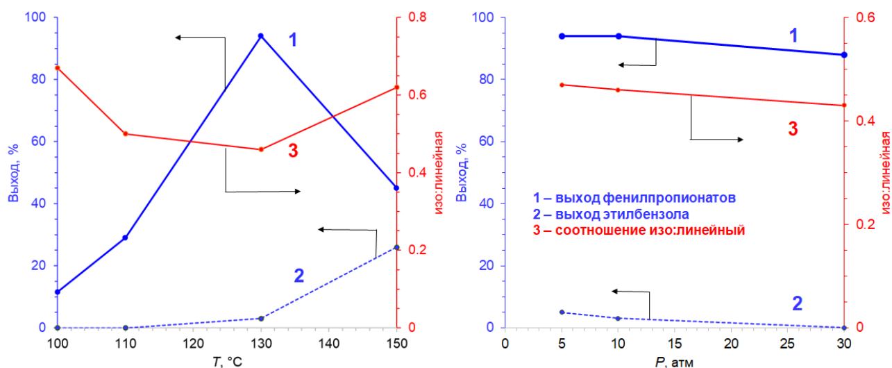
Рис. 1. Влияние температуры (P 10 атм) и давления (T 130°) и на метоксикарбонилирование стирола. Стирол 1.75 ммоль, \text{Ru}_3(\text{CO})_{12} 0.33 мол%, [bmim]Br 200 мол%, MeOH 3 мл, 4 h.
