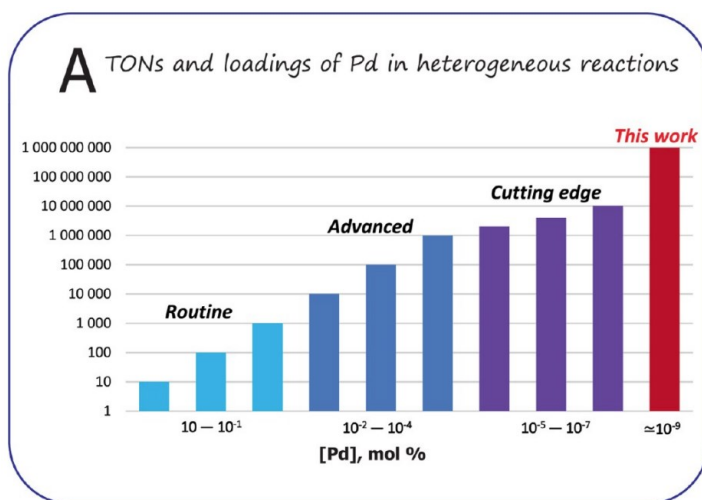
Рисунок 1. Значения TON и загрузки палладиевых катализаторов в гетерогенных каталитических системах [1].
