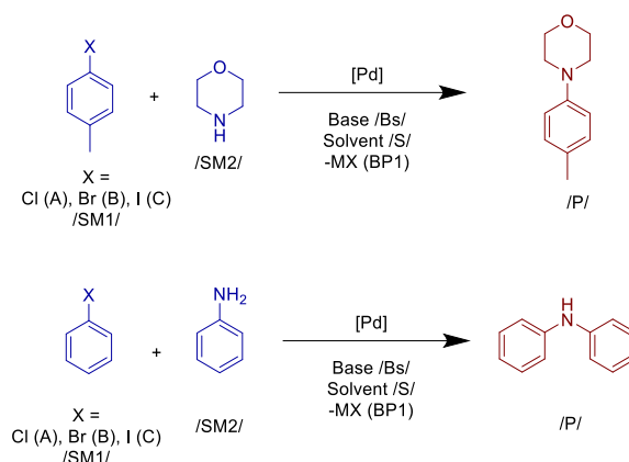
Рис 1. Модельные реакции, охарактеризованные в данной работе.
