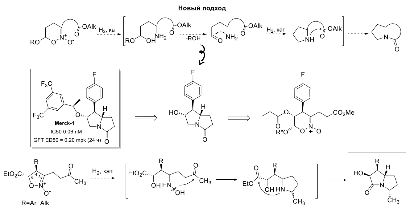
Рис. 1. Домино-стратегия синтеза пирролизидинов
