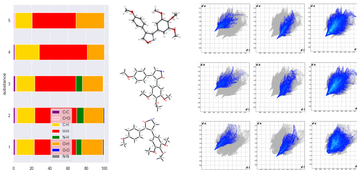
Рис.1. Сравнительная таблица взаимодействий в кристалле у исследуемых соединений.
