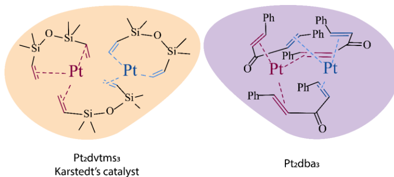
Рис. 1. Структуры катализатора Карстеда и Pt 2 dba 3 .
