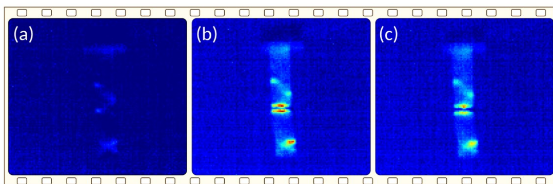
Рис. 1. Термограммы пластикового FFF-образца: (а) до разрушения, (б) в момент разрушения, (с) сразу после разрушения.
