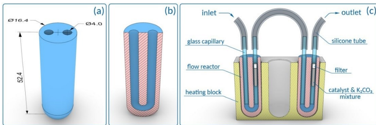
Рис. 1. Проточный реактор для процесса гидрирования дифенилацетилена: (а) 3D-модель реактора с основными размерами (мм); (б) разрез реактора; (с) разрез модульной проточной системы.
