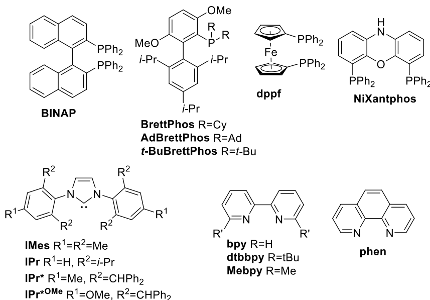
Рис. 1. Типичные примеры P-, NHC- или N-лигандов, используемые в Ni катализе.
