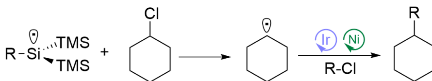
Рис. 1. Схема получения алкильных радикалов.
