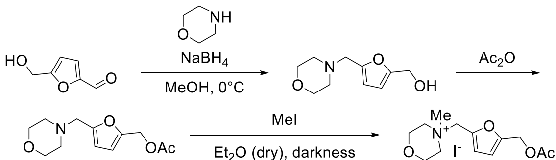
Рис. 1. Схема синтеза.
