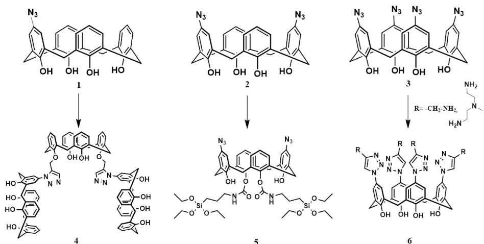
Рис. 1. Синтез азидсодержащих макроциклов и их дальнейшая функционализация.
