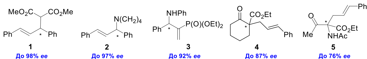
Рис. 2. Результаты каталитических опытов.
