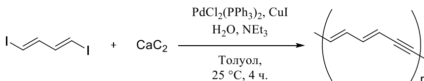
Рис.1. Реакция между 1,4-дидиодбута-1,3-диеном и карбидом кальция.
