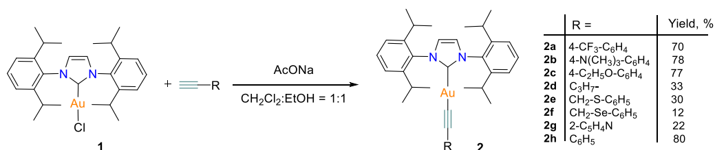
Рис. 1. Общая схема синтеза комплексов NHC/Au (I).
