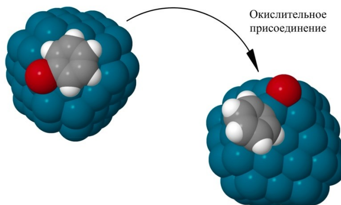
Рис. 1. Каталитический цикл.
