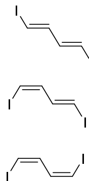
Рис. 2 Изомеры 1,4-дийодбутадиена
