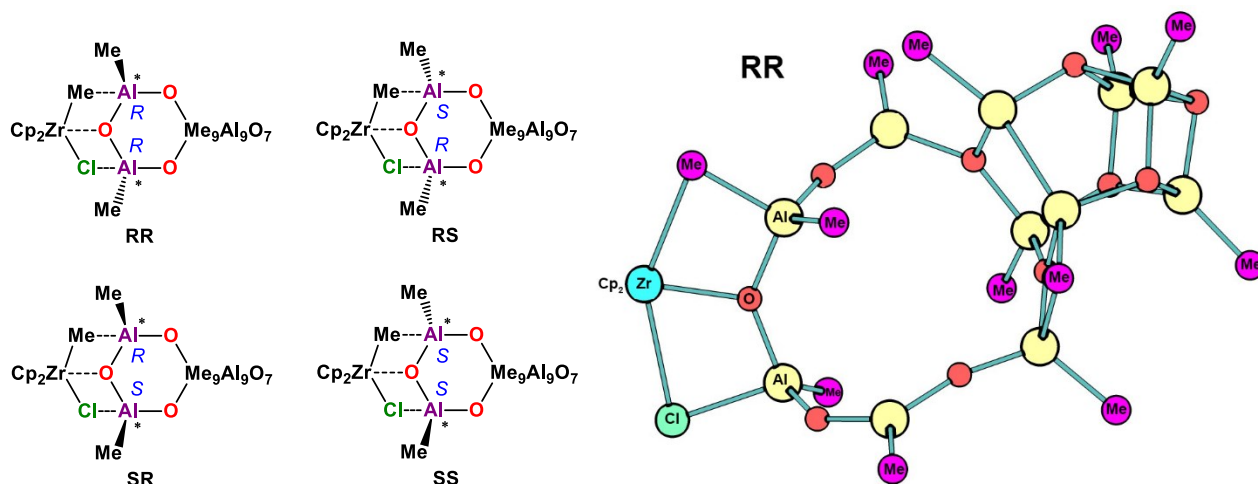
Рис. 1. Диастереомеры комплекса \text{Cp}_2\text{ZrMeCl} с MAO ( \text{Me}_{11}\text{Al}_{11}\text{O}_{10} ).
