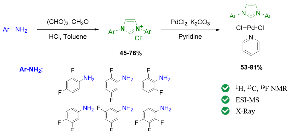
Рис. 1. Схема синтеза Pd/NHC комплексов.
