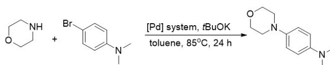
Схема 1. Модельная реакция Бахвальда-Хартвига
