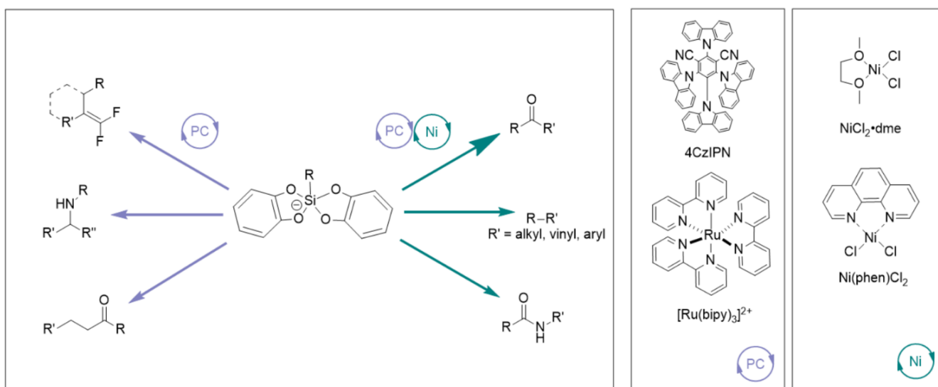
Рис. 4. Схемы реакций с алкилсиликатами.
