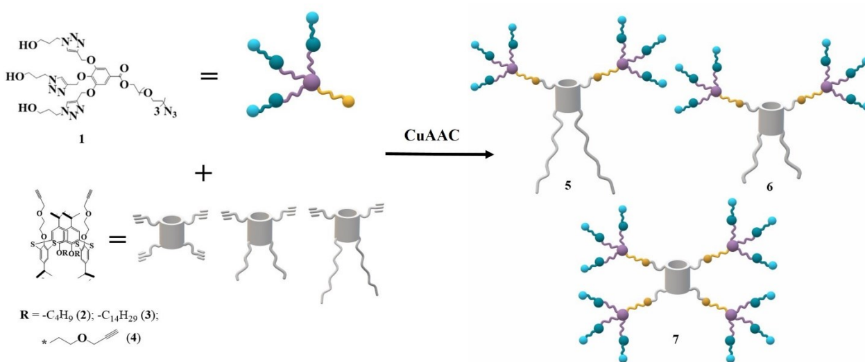
Рис. 1 Получение дендримеров ( 5-7 )
