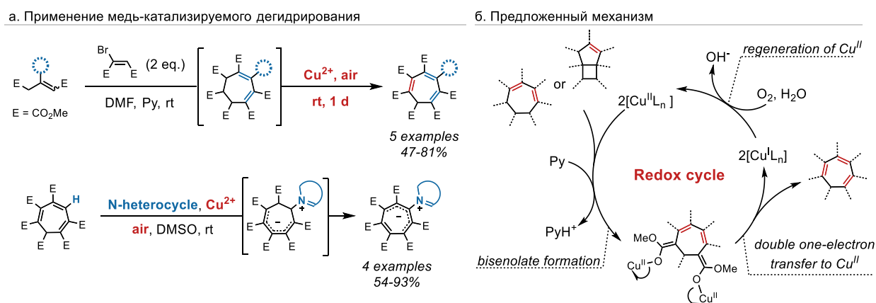
Рис. 1. \text{Cu}^{2+} -катализируемое дегидрирование функционализированных карбоциклов.
