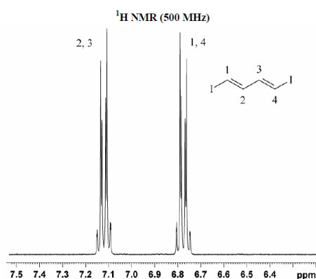
Рис.1 Спектр 1 H-ЯМР 1,4-дийодбутадиена [1]
