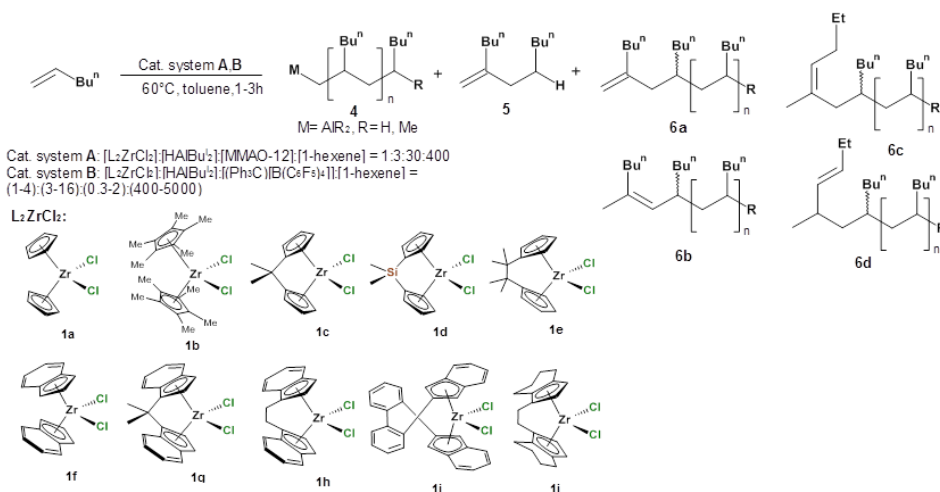
Рис. 1. Трансформация 1-гексена в системе \text{L}_2\text{ZrCl}_2 – АОС – активатор.
