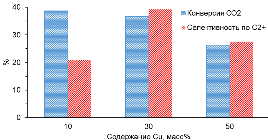
Рис. 1. Влияние содержания Cu на каталитические показатели. Условия: T 200°C, P 10 атм, H 2 :CO 2 = 3, расход газа 2 л ч -1 Γ кат -1 .
