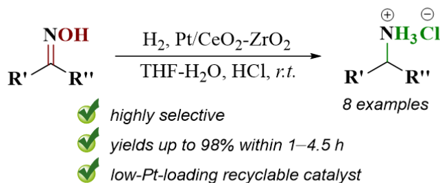
Рис. 1. Схема восстановления оксимов водородом на катализаторе 1%Pt/CeO 2 -ZrO 2
