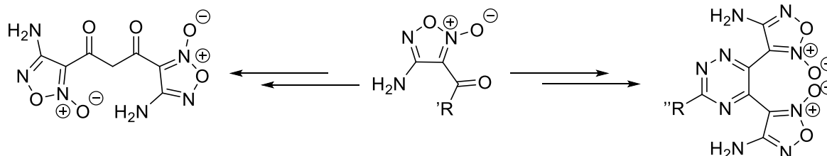
Схема 3. Предложенные синтетические цепочки
