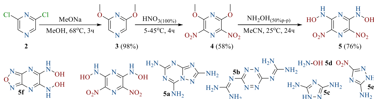
Схема 2. Синтез 2,6-дигидроксиламино-3,5-динитропирозина и молекулярных комплексов на его основе
