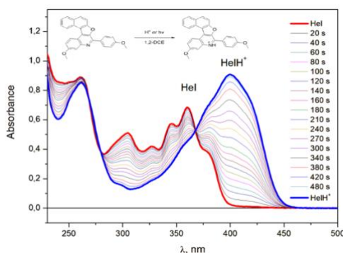
Рисунок 2. Фотопротонирование (308 нм) азагелицена 4 в 1,2-дихлорэтано.
