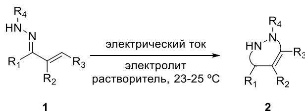
Схема 1. Электрохимическая реакция
