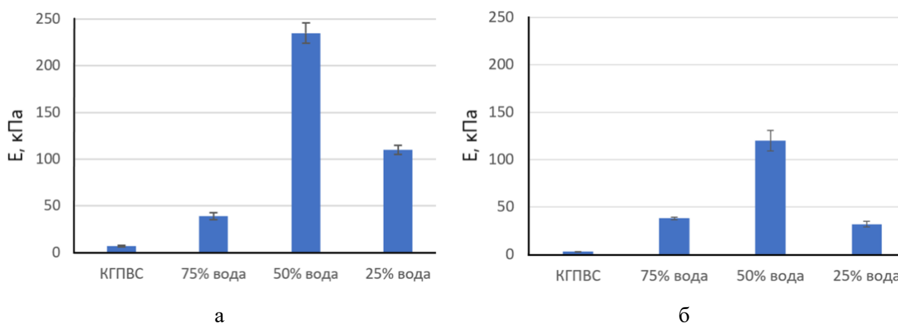
Рис.1 Зависимости модуля Юнга КГПВС от соотношения H_2O /ДМСО для КГПВС, полученных из водного (а) и ДМСО (б) 10% раствора полимера.
